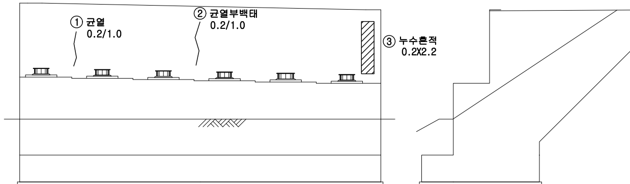
정면
